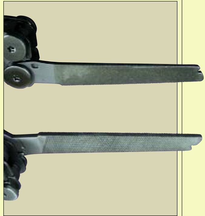
Наче следует раскрыть рукоятки, а только затем доставать отвертки. Напильник Wave (фото с обеих сторон)
